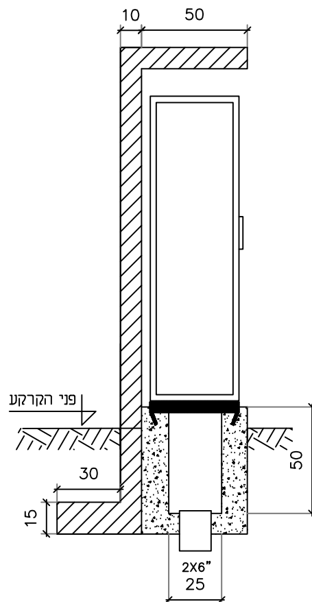
חתך ג-ג (צד)
