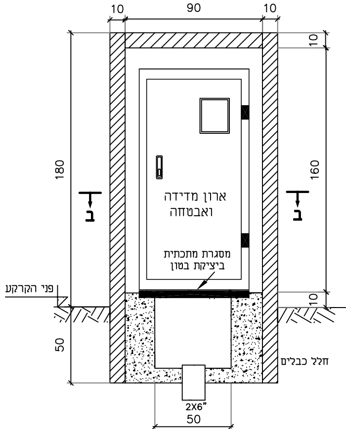
חתך א-א (חזית)
